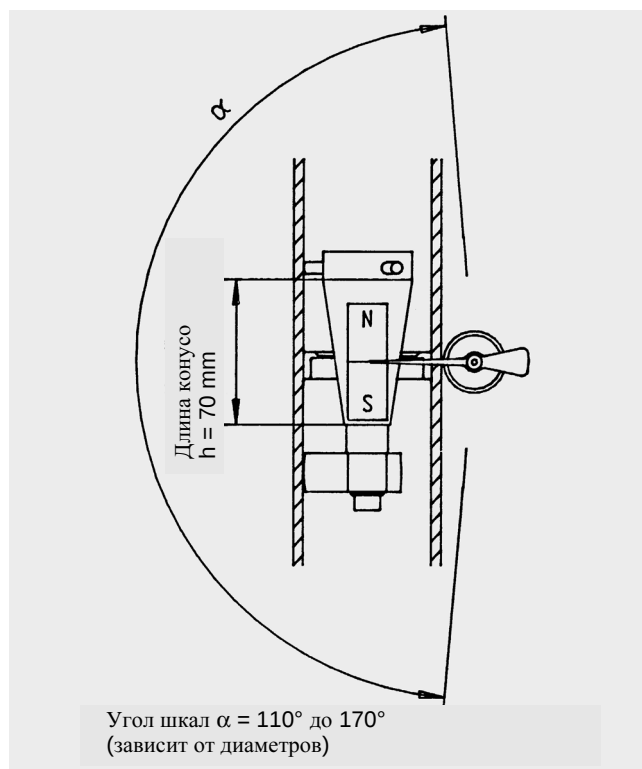
Рис 3/88 Измерительный конус/угол шкал
