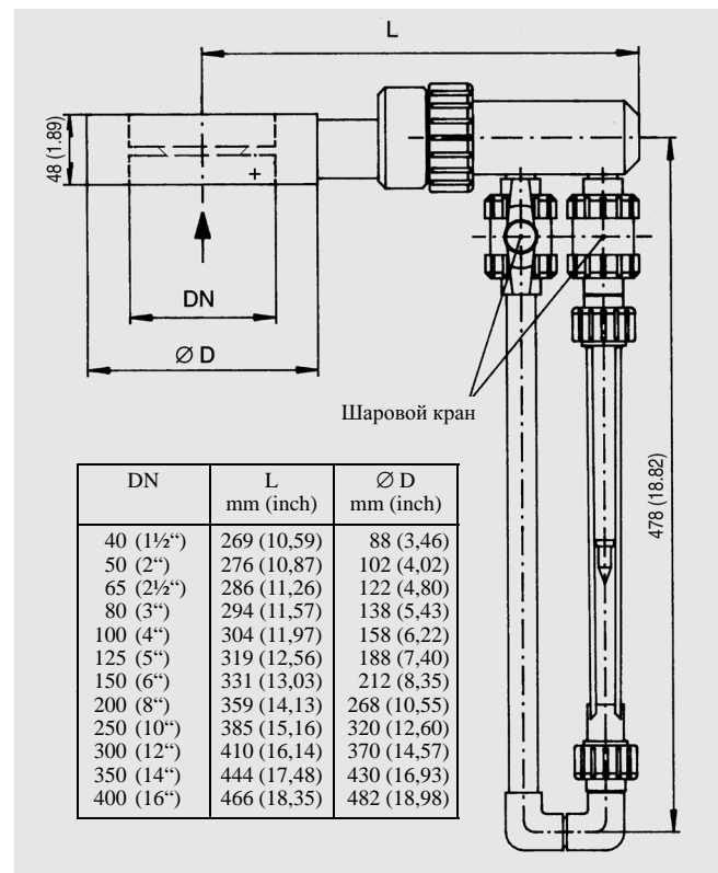
Рис 3/102 SITRANS FO N4, размеры в мм (inch)
