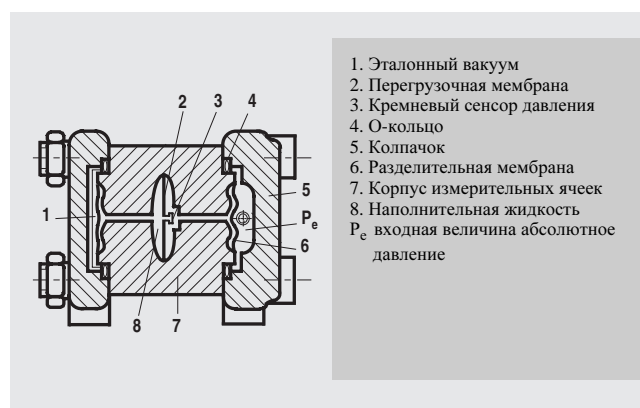
Рис 1/35 Измерительная ячейка для абсолютного давления из серии "Дифференциальное давление", функциональная схема
