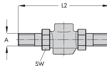
Резьбовое соединение с патрубками под резьбу
