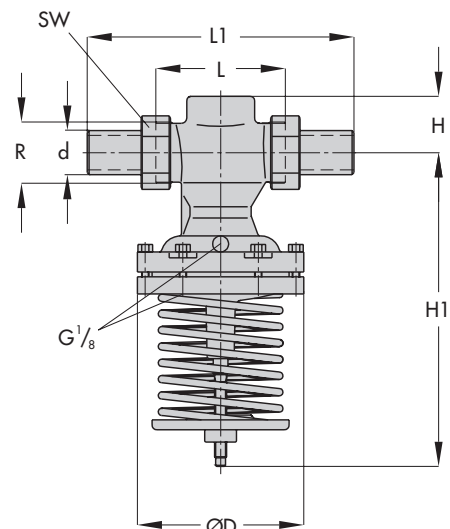
Резьбовое соединение с патрубками под сварку тип 45-6
