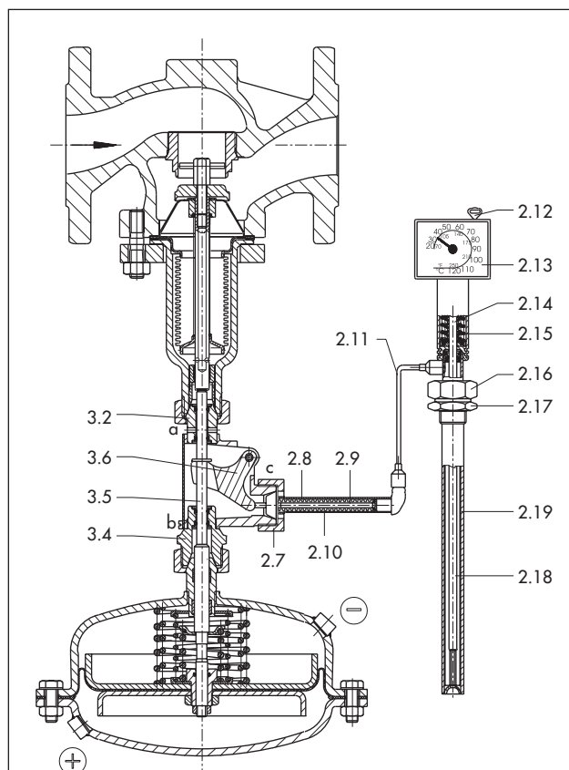
Рис. 3 · Регулятор перепада давления и температуры тип 42-28 DoT с установочным клапаном тип 2422, двойным подводом и регулирующим термостатом тип 2231
