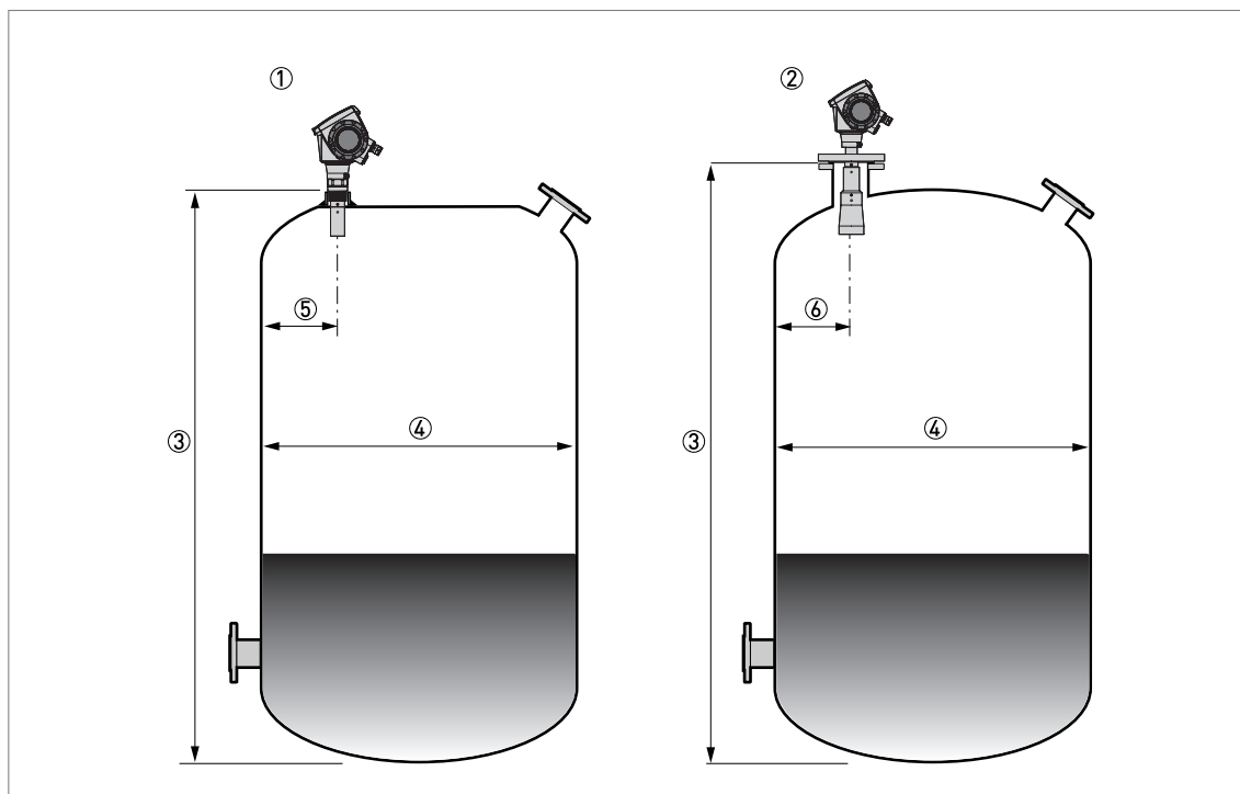
Рисунок 3-1: Рекомендуемое расположение патрубка для жидкостей, паст и суспензий
