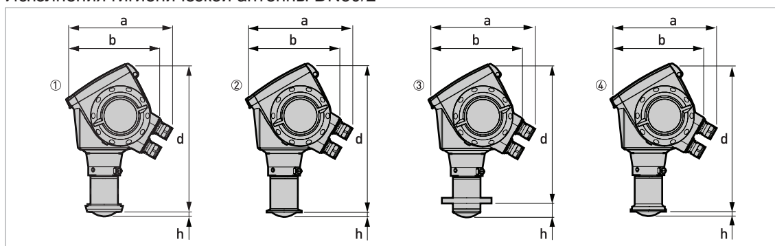
Рисунок 2-16: Исполнения гигиенической антенны DN50/2"
