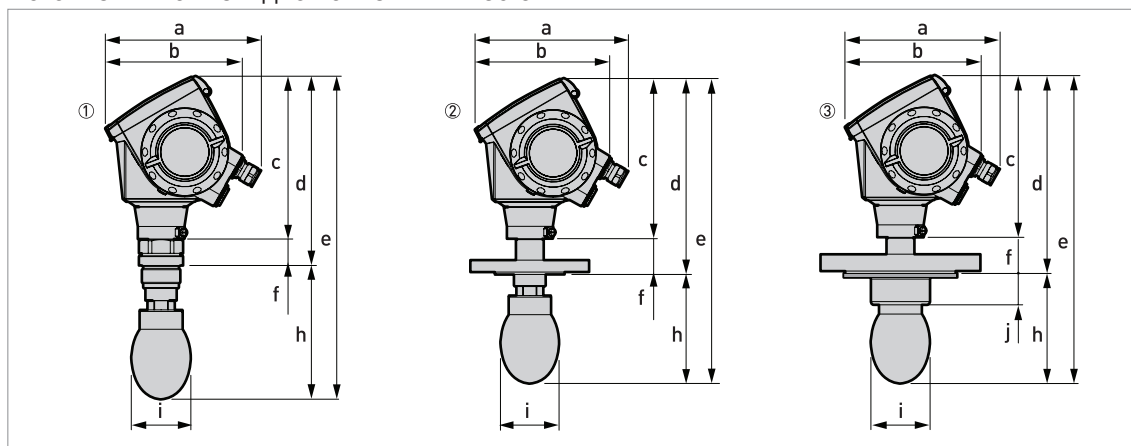
Рисунок 2-14: Исполнения каплевидной антенны DN80/3"
