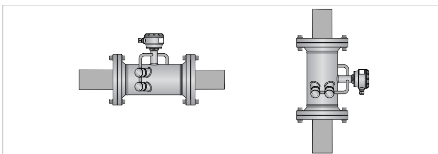
Рисунок 3-4: Монтаж в горизонтальном и вертикальном положении
