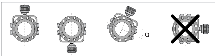
Рисунок 3-3: Монтажное положение прибора
