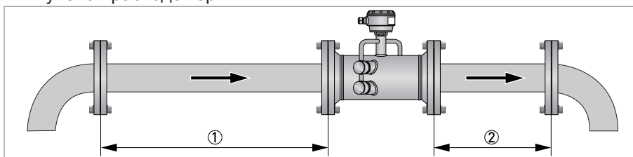
Рисунок 3-2: Рекомендуемые длины прямых участков на входе и выходе прибора для \geq \text{DN}100/4 дюйма
