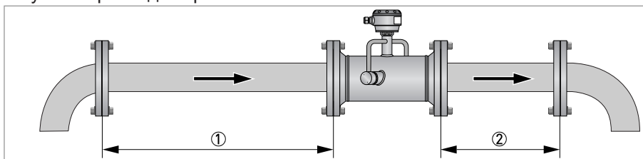
Рисунок 3-1: Рекомендуемые длины прямых участков на входе и выходе прибора для \leq \text{DN}80/3 дюйма
