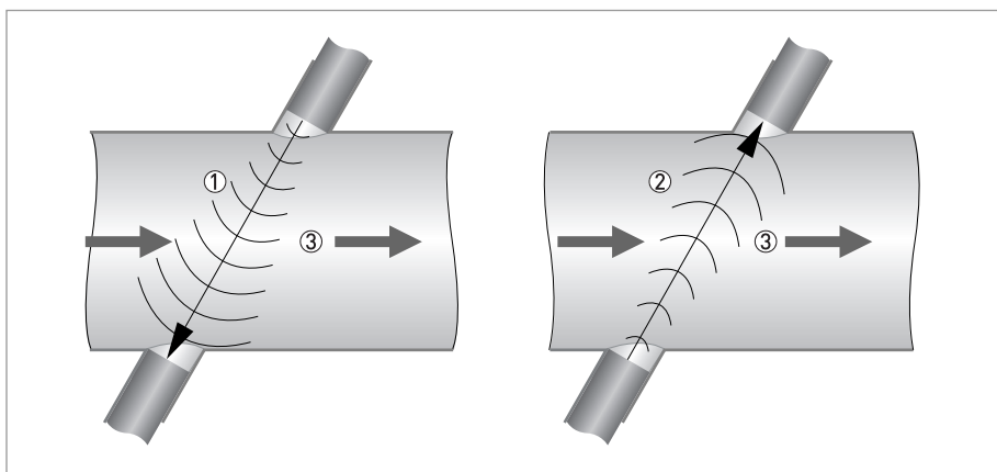
Рисунок 1-1: Принцип измерения
