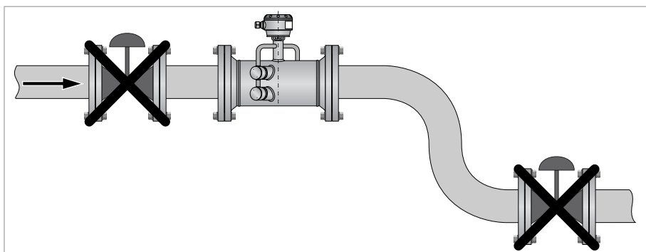
Рисунок 3-8: Наличие регулирующего клапана
