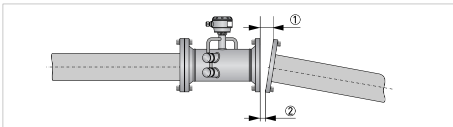
Рисунок 3-5: Несоосность фланцевых соединений
