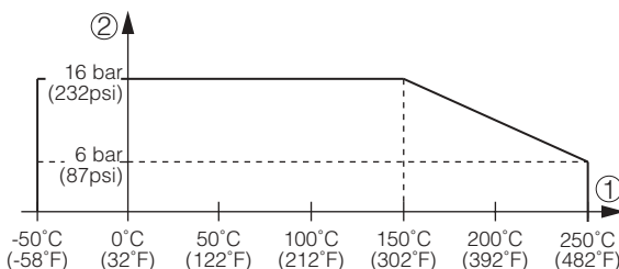
Рис. 17: Давление процесса - Температура продукта
