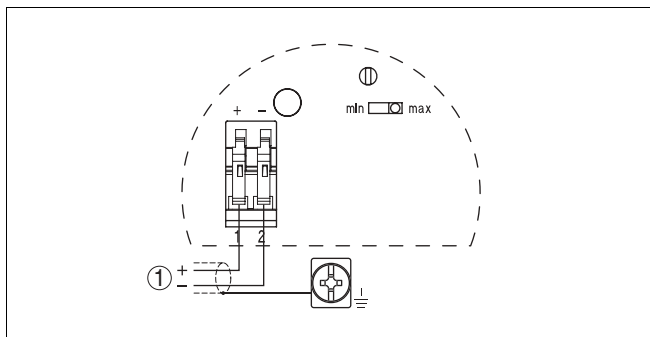
Рис. 11: Схема подключения
