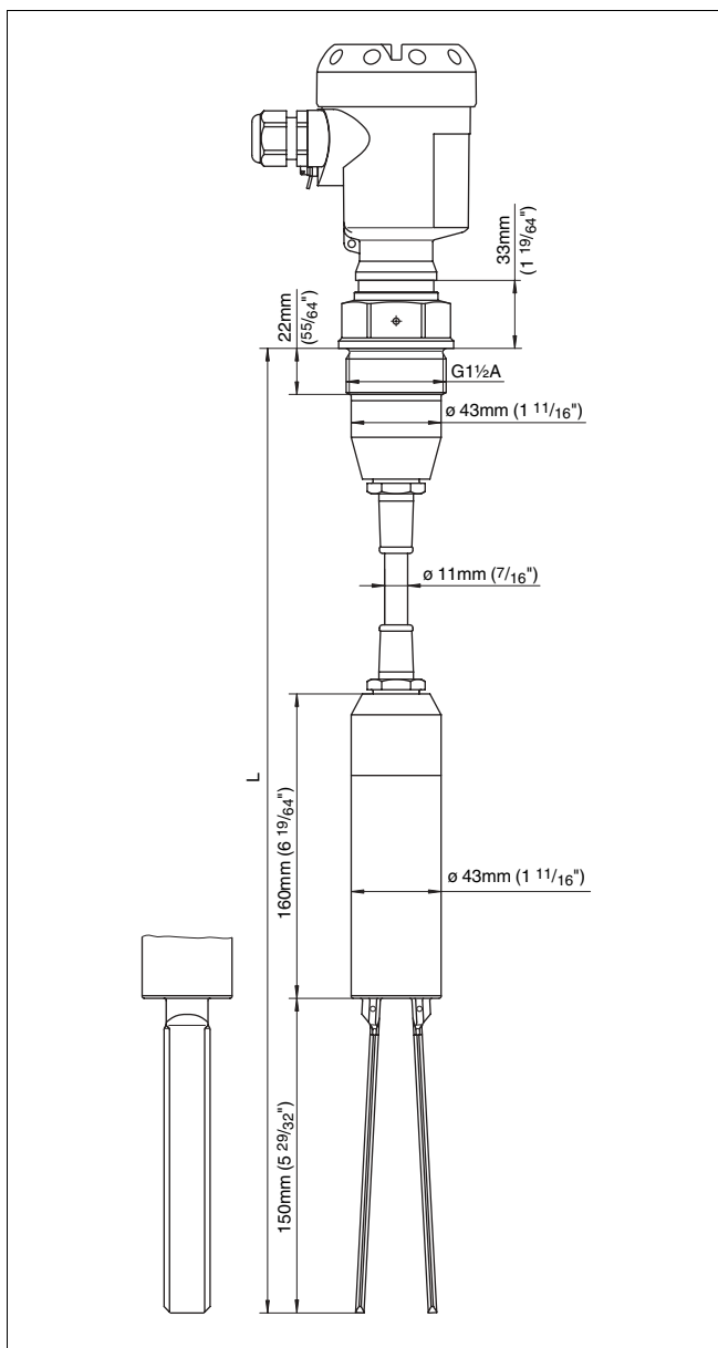
Рис. 18: OPTISWITCH 3200 C с резьбовым присоединением G1 1/2 A L = Длина датчика, см. Технические данные
