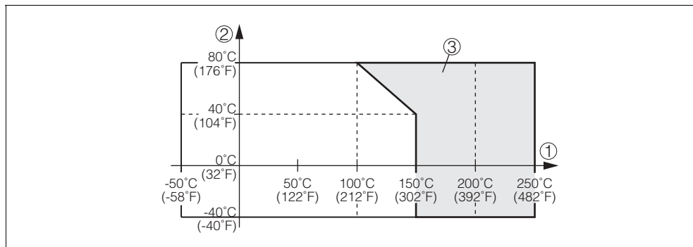
Рис. 15: Температура окружающей среды - Температура продукта
