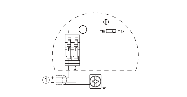
Рис. 10: Схема подключения
