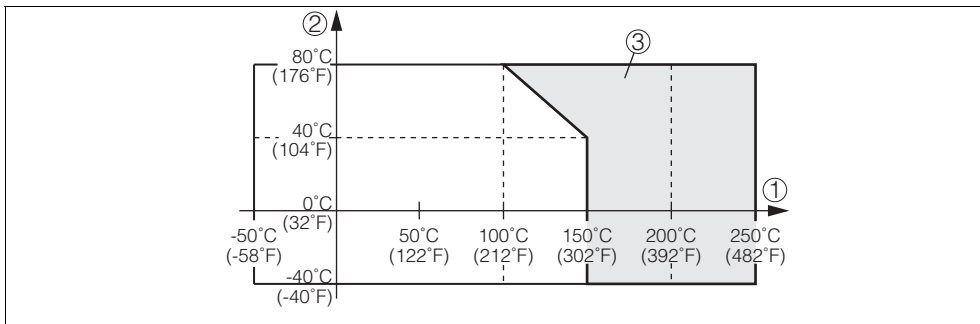
Рис. 15: Температура окружающей среды - Температура продукта
