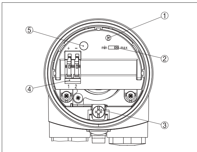
Рис. 11: Блок электроники VB 60Z - двухпроводный выход
