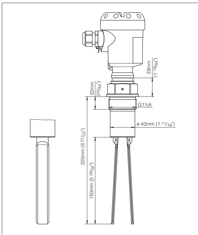
Рис. 17: OPTISWITCH 3100 C с резьбовым присоединением G1 1/2 A
