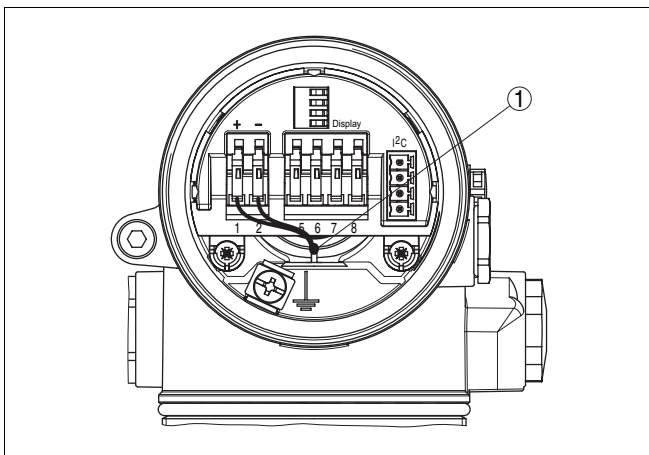
Рис. 17: Отсек электроники в двухкамерном корпусе
