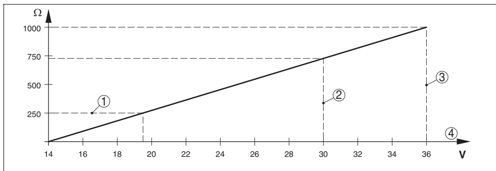
Рис. 26: Диаграмма напряжения
