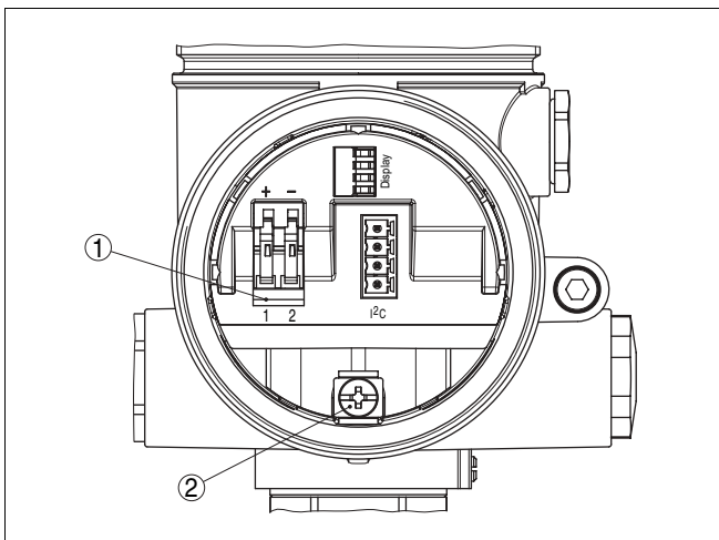
Рис. 21: Отсек подключения в двухкамерном корпусе
