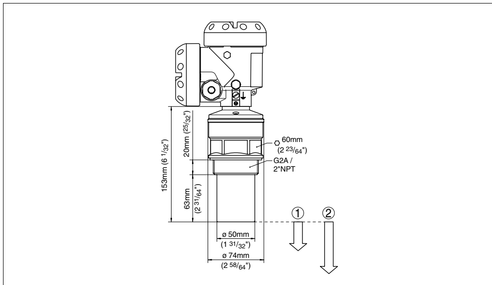
Рис. 23: OPTISOUND 3020 C
