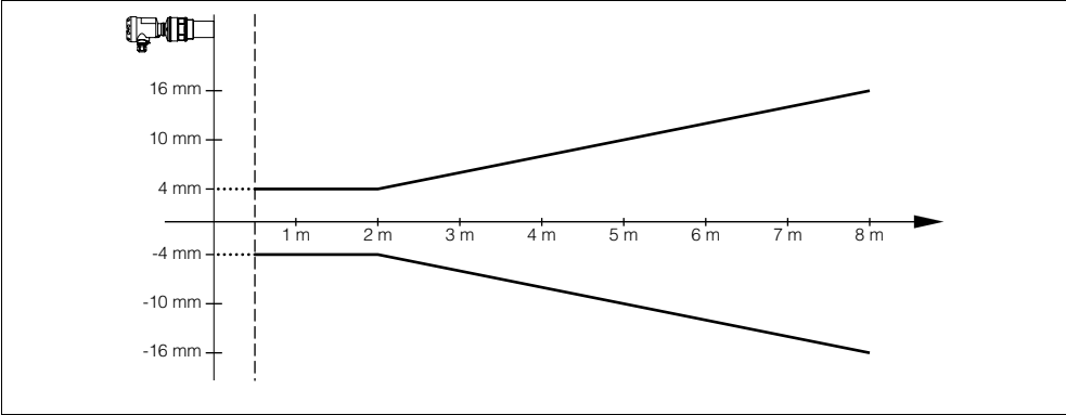
Рис. 22: Точность OPTISOUND 3020 C
