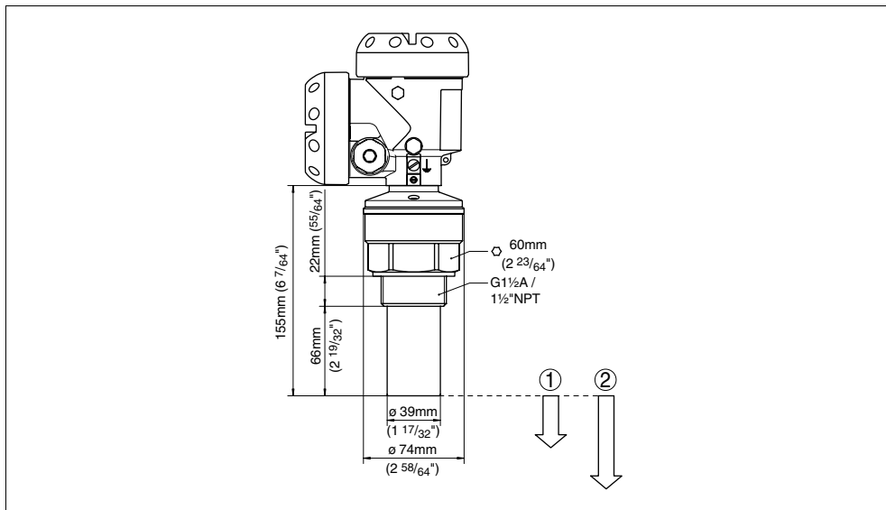
Рис. 23: OPTISOUND 3010 C
