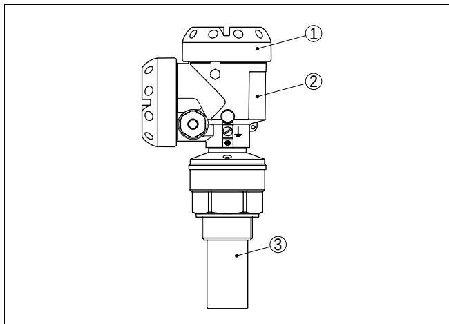
Рис. 1: OPTISOUND 3010 C с алюминиевым двухкамерным корпусом
