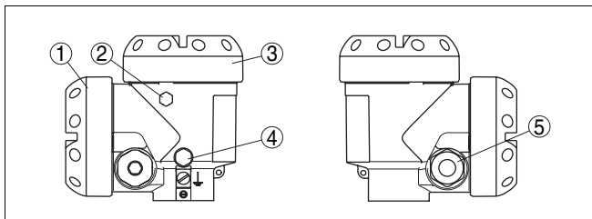
Рис. 16: Двухкамерный корпус
