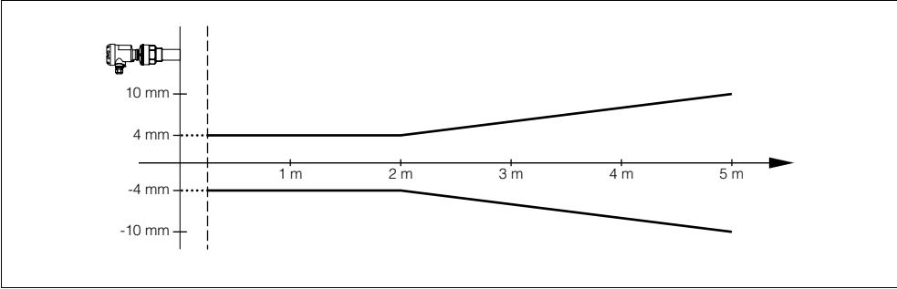
Рис. 22: Точность OPTISOUND 3010 C
