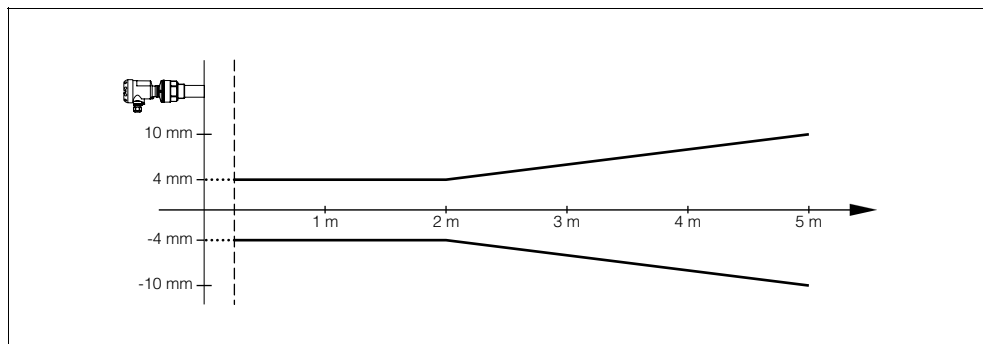
Рис. 25: Точность OPTISOUND 3010 C
