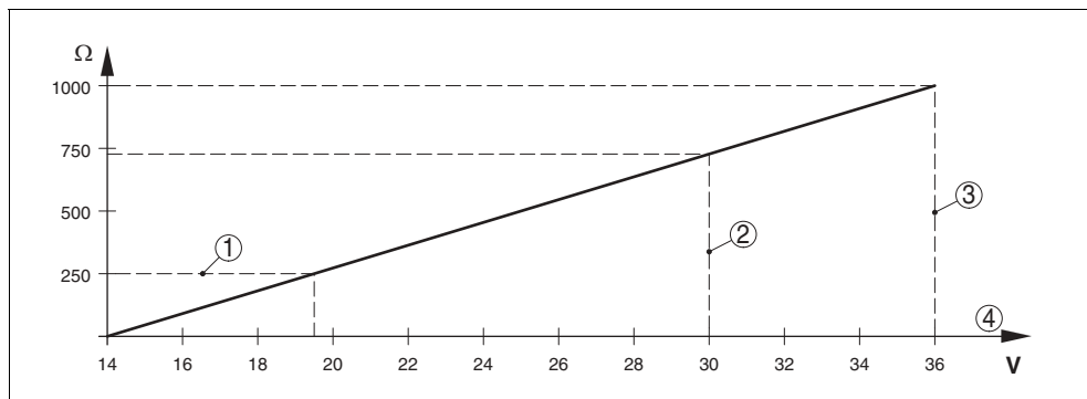
Рис. 26: Диаграмма напряжения
