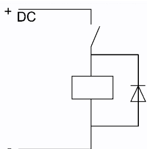
Диод, включенный противоположно к полярности цепи питания
