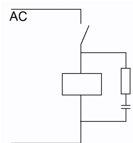
RC – цепь
